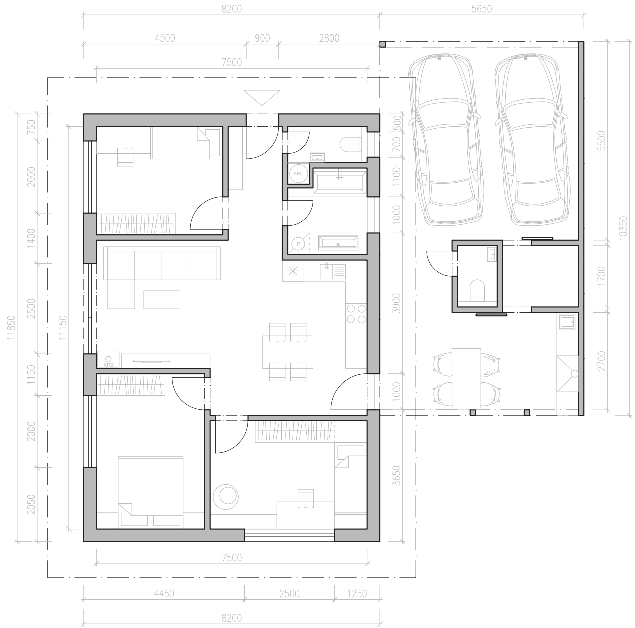
PŮDORYS DOMU
